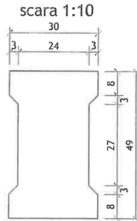
PLACUȚĂ CAROSABILĂ DIN BETON ARMAT
