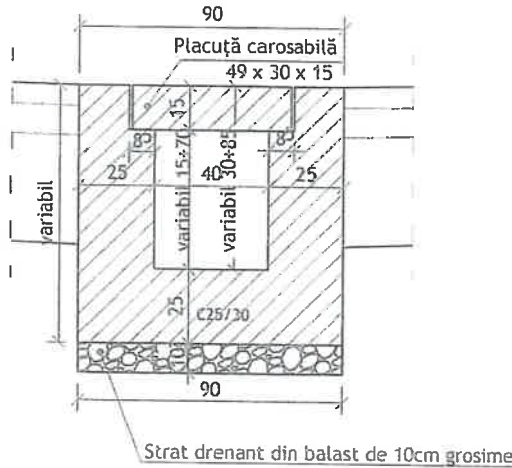
SECȚIUNE TRANSVERSALĂ scara 1:20
